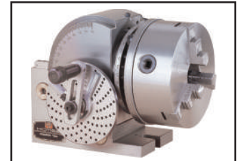
Acessórios Opcionais: Placa de 3 castanhas 6".
