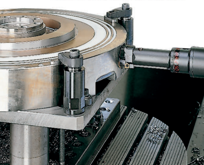
Fig. 3 – Os cabeçotes de mandrilhamento são ajustados com a possibilidade de utilizar somente uma cápsula, para operações de desbaste e acabamento com remoção leve de material. A placa de proteção para o serrilhado deve sempre ser usada para este tipo de operação.
