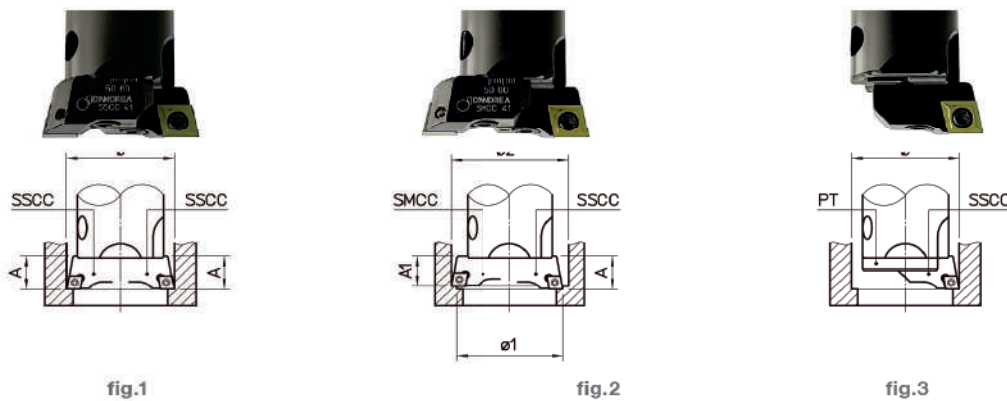
Fig. 1 – Na utilização de duas cápsulas SSCC usinando juntas, ajustadas na mesma distância radial para operações de desbaste de alta velocidade.
