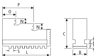
Castanhas Monobloco Interna
