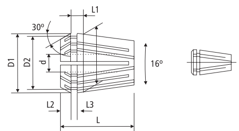
ER11 - ER50
