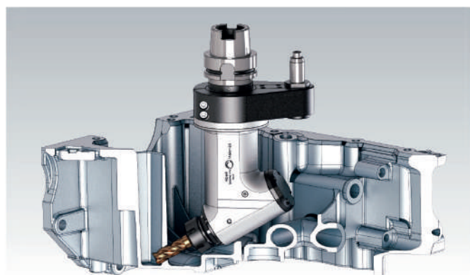
Cabeçote fixo com ângulo variável
