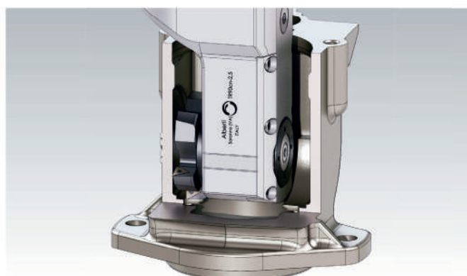
Cabeçote para espaços restritos
