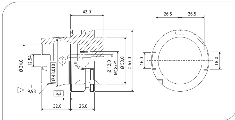
HSK - A63
