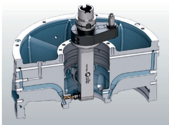
Cabeçote 90° longo
